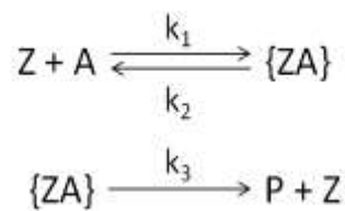
Figura 2 – Reacciones químicas de la detoxificación por agregado de \text{Ca}(\text{OH})_2
