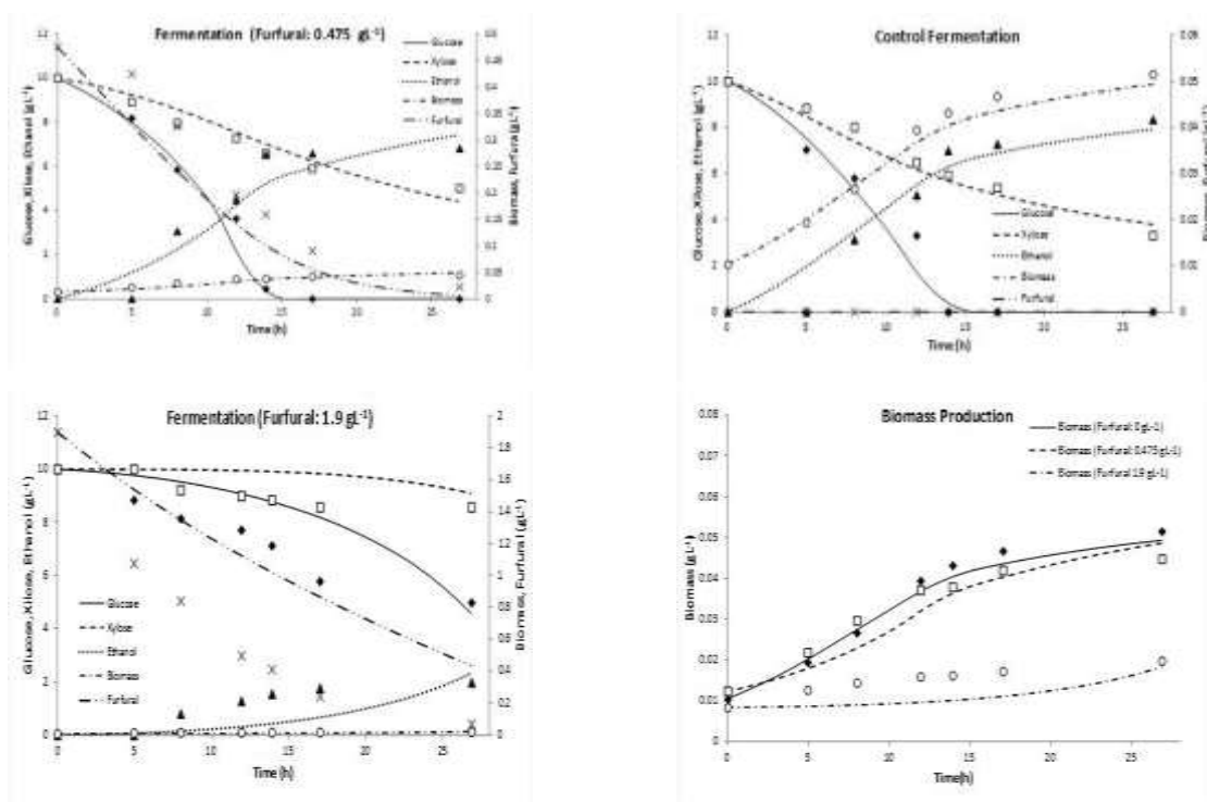
Figura 3 – Perfiles óptimos de concentración vs datos experimentales para glucosa(♦), xilosa(□), etanol(▲), biomasa(○) y furfural(X)
