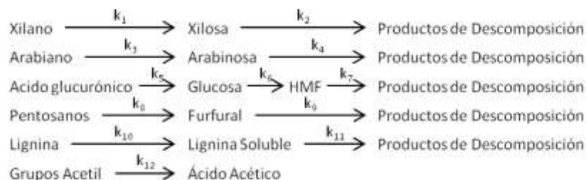
Figura 1 – Reacciones químicas de la hidrólisis ácida
