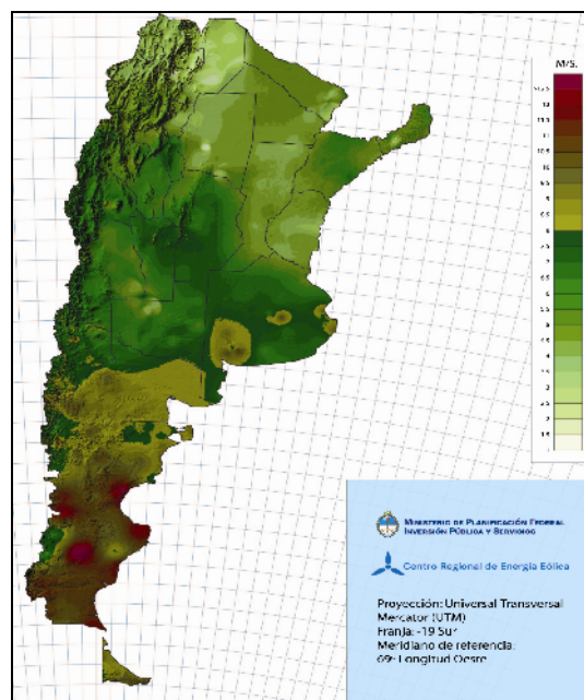
Figura 4 – Mapa de Velocidad Media anual del viento a 50 m de altura
