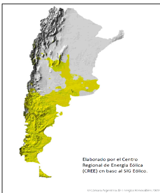
Figura 3 – Mapa de zonas con factor de capacidad mayor a 35% a 70 m de altura
