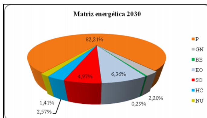
Figura 5 – Matriz energética Escenario A, al año 2030
